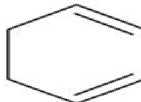
1,3 - cyclohexadiene
