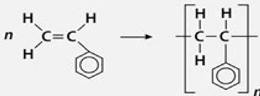
Styrene
