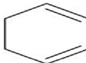
1,3 - cyclohexadiene
