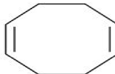
1,5-Cyclooctadiene
