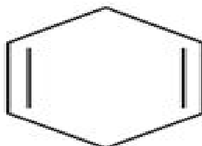
1,4 - cyclohexadiene
