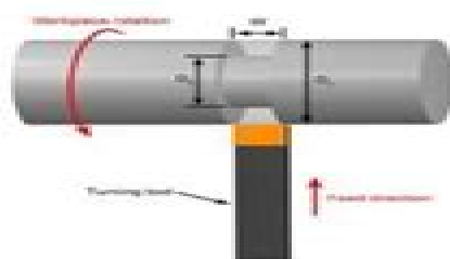
Grooving
