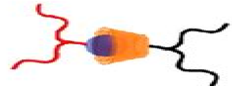
miktoarm star
