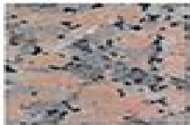
Granodiorite
