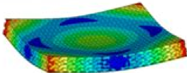
Mode 3: 3389.8 Hz.
