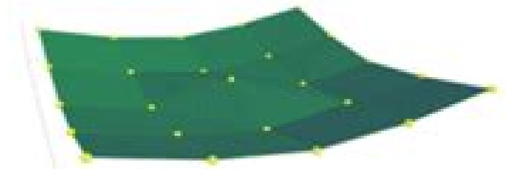
Mode 3: 3221.2 Hz.
