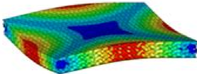
Mode 2: 2781.5 Hz.
