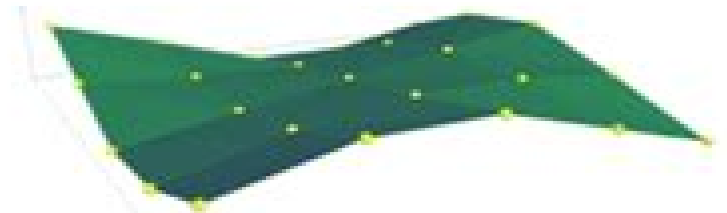
Mode 2: 2636.7 Hz.
