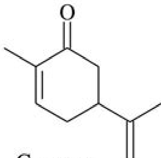
Carvone
